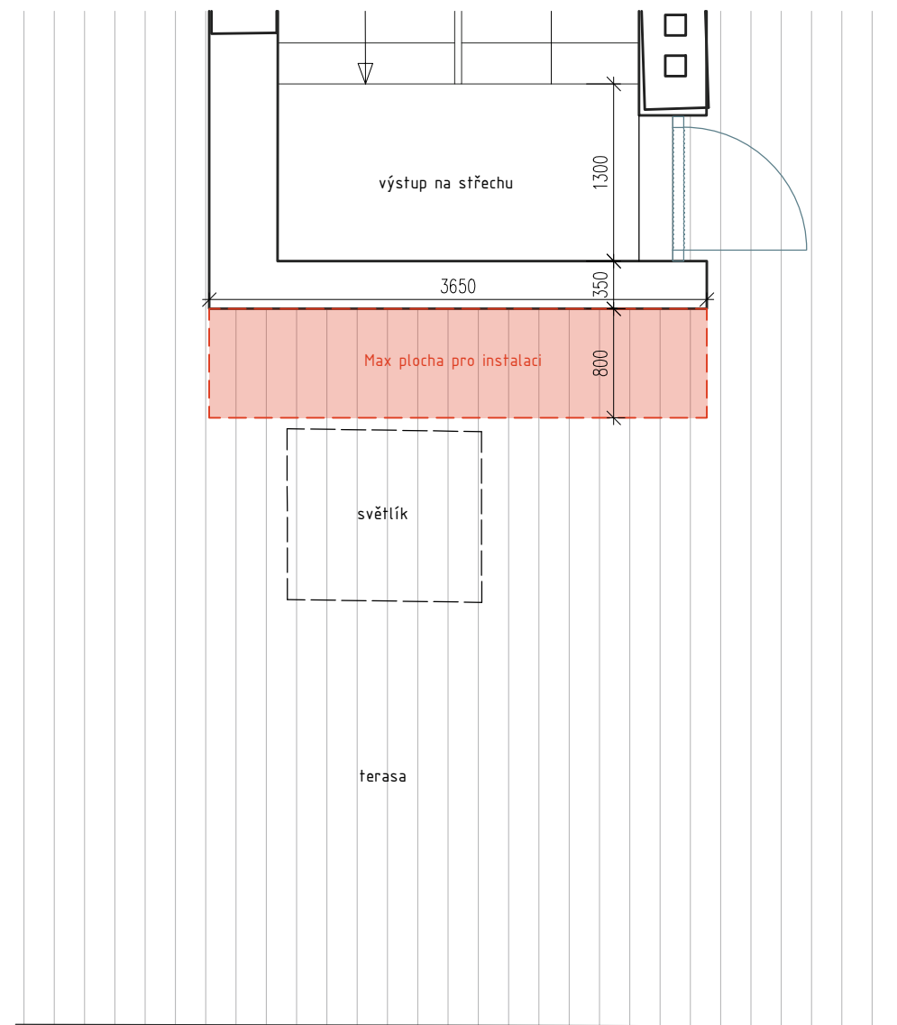
PŮDORYS
